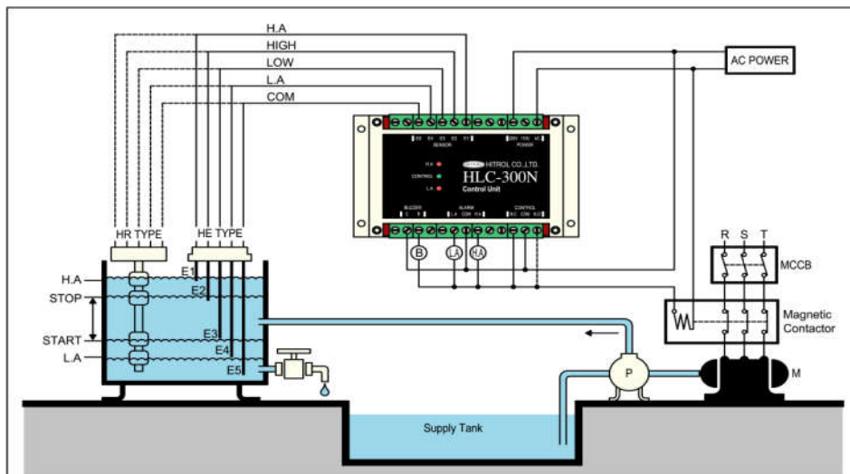
<HLC-300N>
